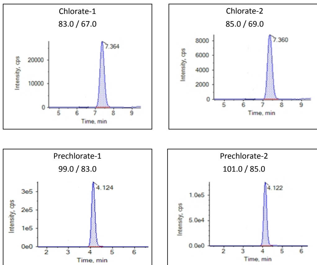
图A.1 氯酸盐、高氯酸盐特征离子色谱图 (100mm×2.1mm, 3 \mu m 规格色谱柱)
