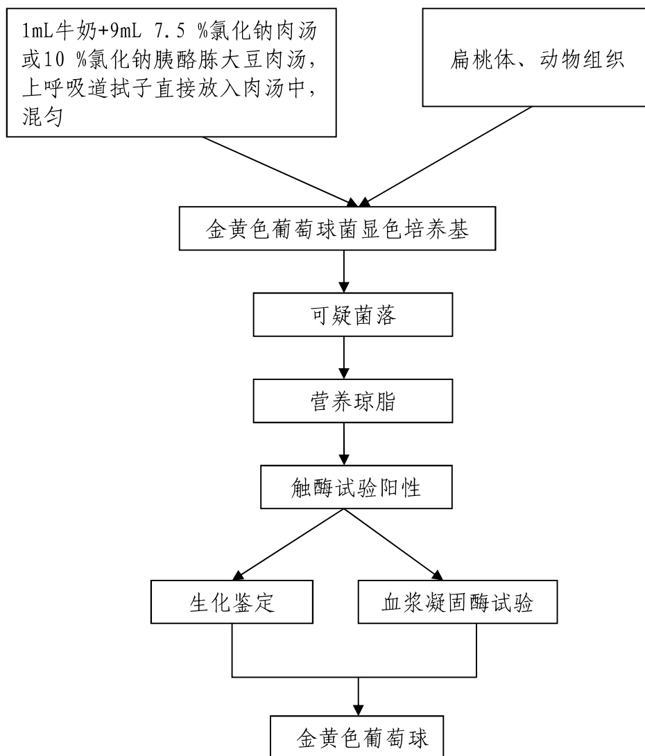
图3 金黄色葡萄球菌分离和鉴定程序
