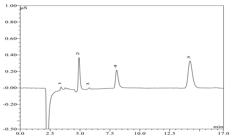
图10 沙尘气溶胶样品中水溶性阴离子色谱图 (1- F - 、2- Cl - 、3-NO 2 - 、4-NO 3 - 、5- SO 4 2- )
