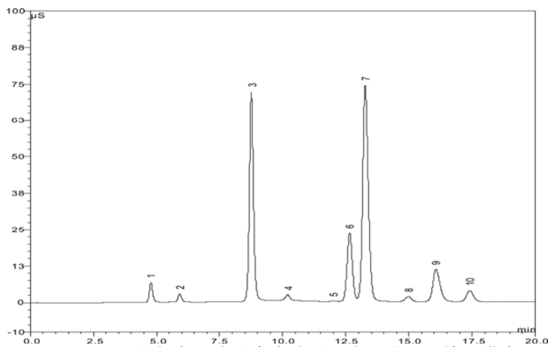
图 8 大气自然降尘中水溶性阴离子谱图 (使用梯度) (1- F - 、2- 乙酸和甲酸、3- Cl - 、4- NO 2 - 、5- CO 3 2- 、6- SO 4 2- 、7- Br - 、8- NO 3 - 、9- PO 4 3- )
