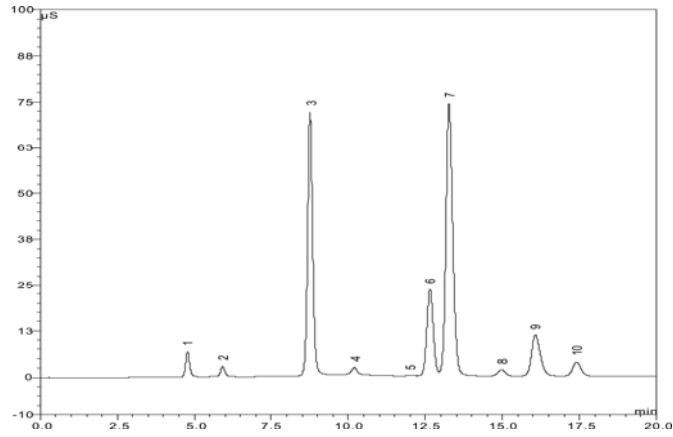
图3 使用梯度淋洗得到的10种阴离子分析谱图 (1-F - 、2-乙酸和甲酸、3-Cl - 、4-NO 2 - 、5-CO 3 - 、6-SO 3 2- 、7-SO 4 2- 、8-Br - 、9-NO 3 - 、10-PO 4 3- )
