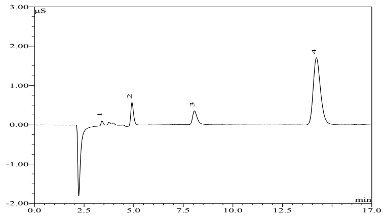
图5 大气颗粒物(PM 10 )样品中水溶性阴离子色谱图 (1-F - 、2-Cl - 、3-NO 3 - 、4-SO 4 2- )
