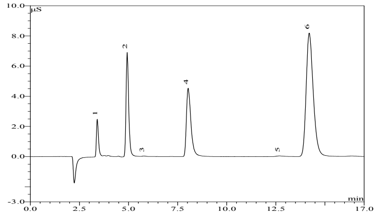
图4 大气颗粒物(TSP)样品中水溶性阴离子色谱图 (1-F - 、2-Cl - 、3-NO 2 - 、4-NO 3 - 、5-SO 3 2- 、6-SO 4 2- )
