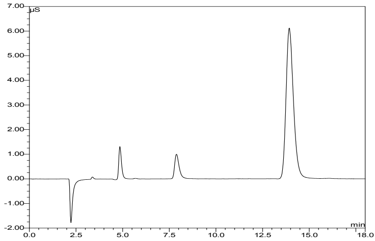
图 6 大气颗粒物 (PM 2.5 ) 样品中水溶性阴离子色谱图 (1- F - 、2- Cl - 、3- NO 3 - 、4- SO 4 2- )
