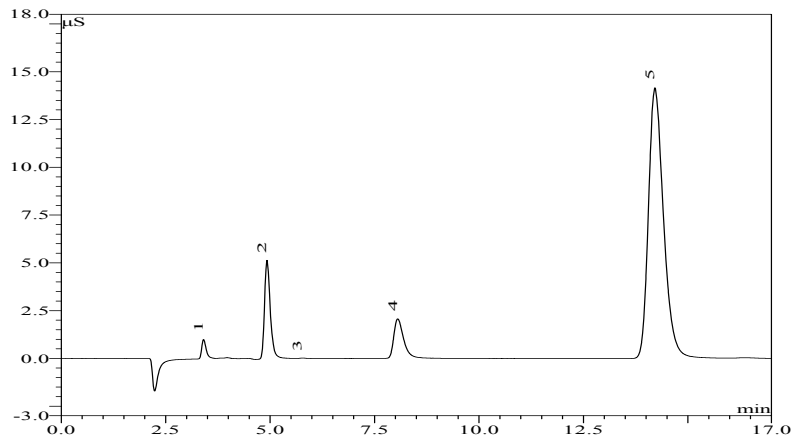
图 7 大气自然降尘样品中水溶性阴离子色谱图 (1- F - 、2- Cl - 、3- NO 2 - 、4- NO 3 - 、5- SO 4 2- )
