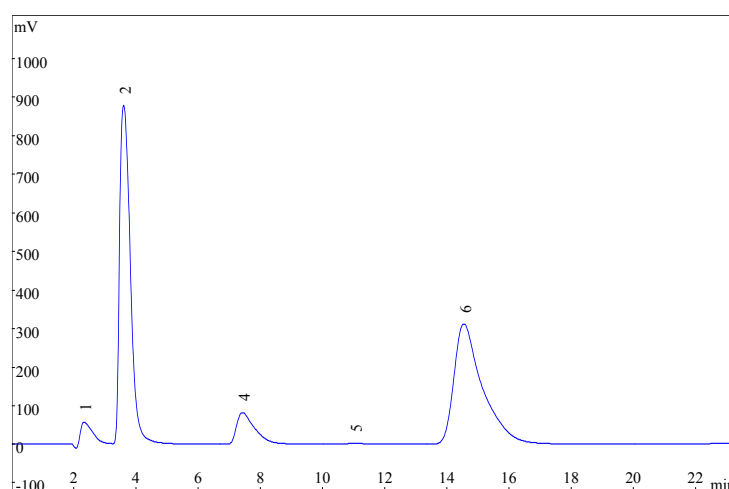
图9 用大气干湿沉降物在线自动监测装置采集和分析的降尘阴离子色谱图 (1- F - 、2- Cl - 、3- NO 2 - 、4- NO 3 - 、5-PO 4 3- 、6- SO 4 2- )
