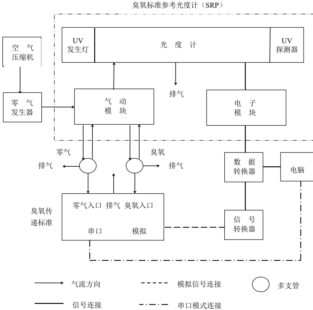
图 2 臭氧监测一级校准管路与信号连接图
