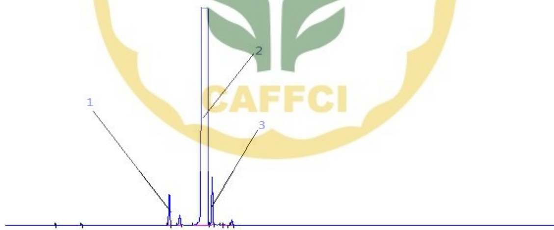
图A.1 食品添加剂 \beta -蒎烯典型气相色谱图
