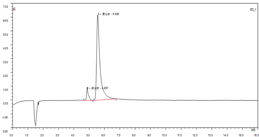
图C.1 氰化物标准离子色谱图（浓度0.02 mg/L）
