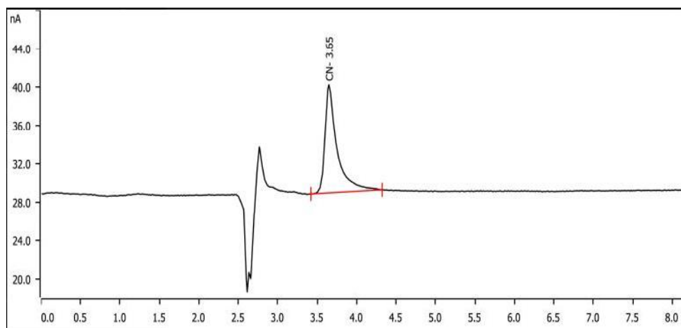
图C. 2 氰化物标准离子色谱图（浓度0.02 mg/L）
