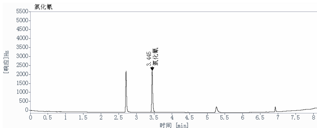
图B.1 氯化氰标准气相色谱图（浓度0.05 mg/L）
