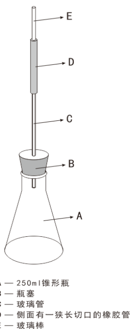
图1 本生阀装置示意图
