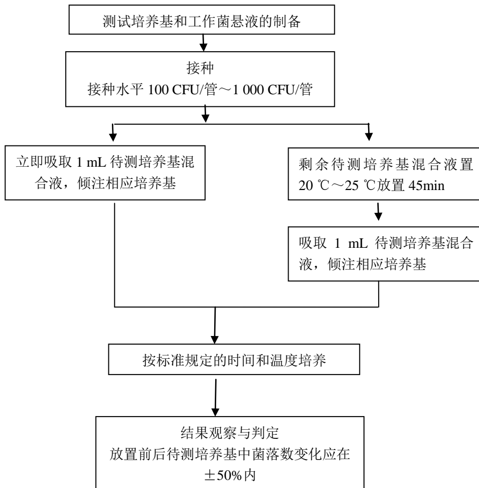
图 A.7 悬浮培养基和运输培养基的定量测定方法流程图
