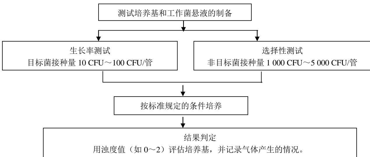
图 A.6 选择性液体计数培养基的半定量测定方法流程图
