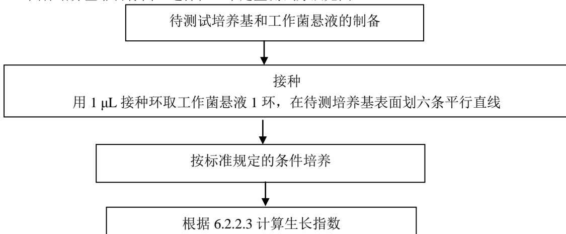
图 A.2 固体培养基非目标菌（选择性）半定量测定方法流程图
