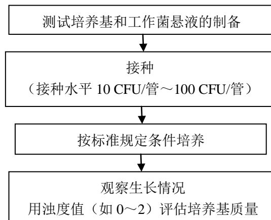
图 A.4 非选择性增菌培养基半定量测定方法流程图
