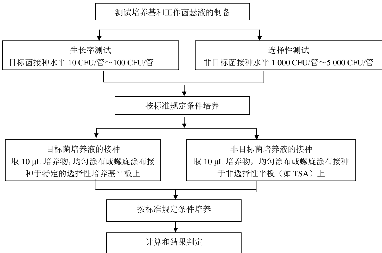
图 A.5 选择性增菌培养基的半定量测定方法流程图
