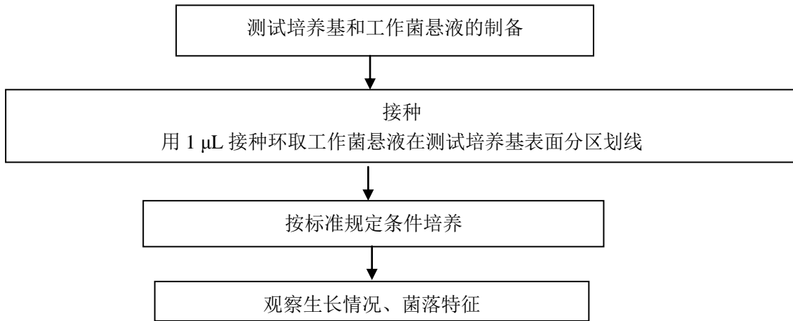
图 A.3 固体培养基非目标菌（特异性）定性测定方法流程图
