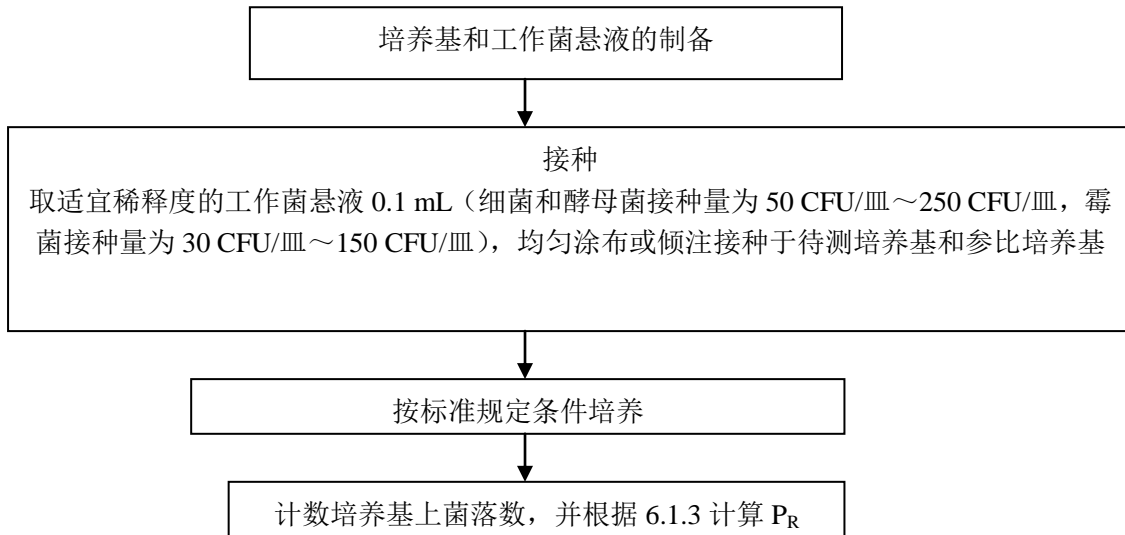
图 A.1 固体培养基目标菌生长率定量测定方法流程图
