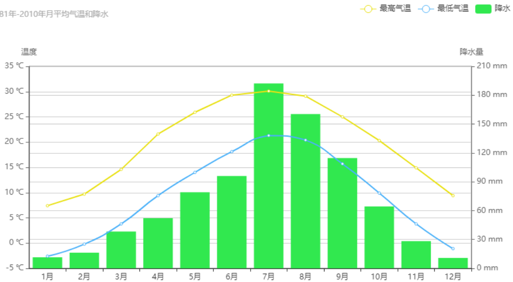
商洛市商南县 1981-2010 年月平均气温及降水情况
