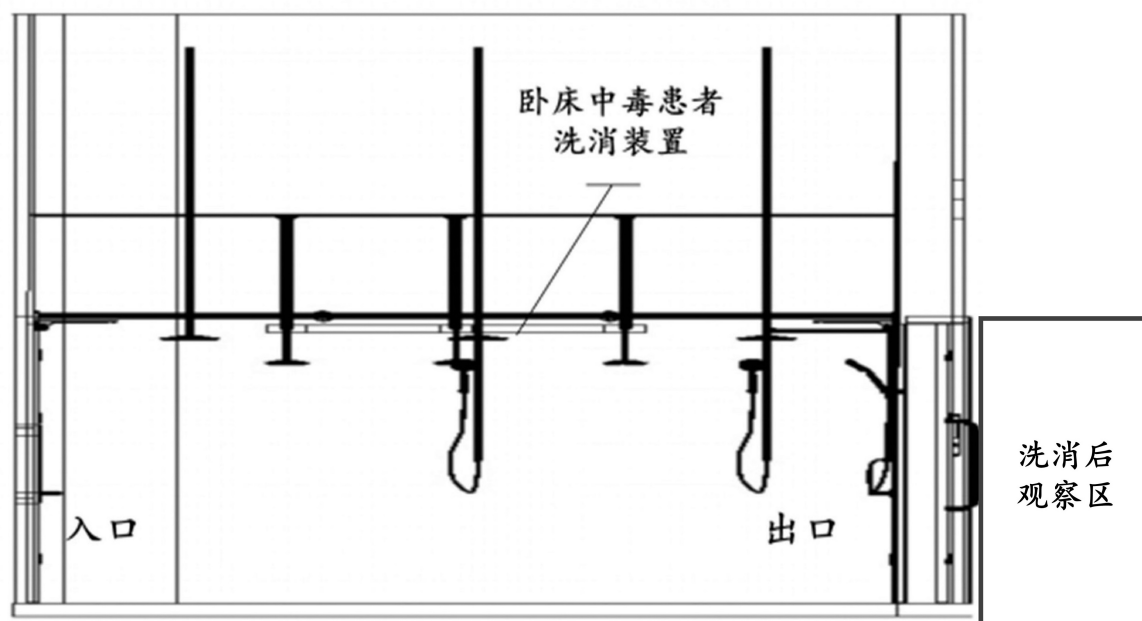
图 A. 3 患者洗消单元模式图
