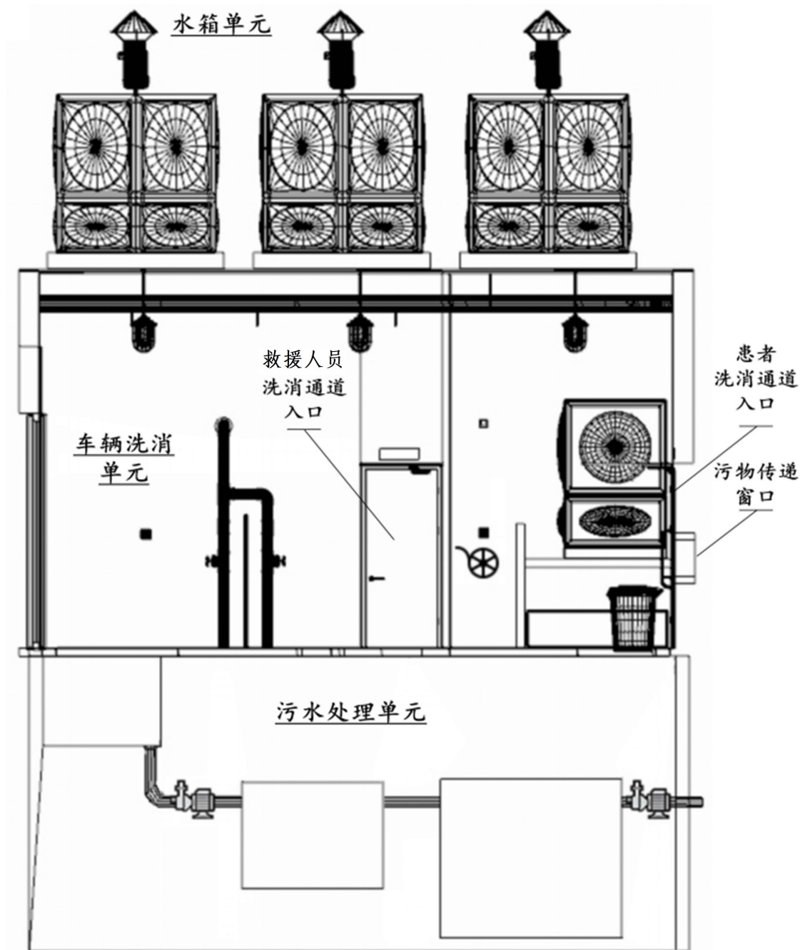
图 A.1 水路设计模式图
