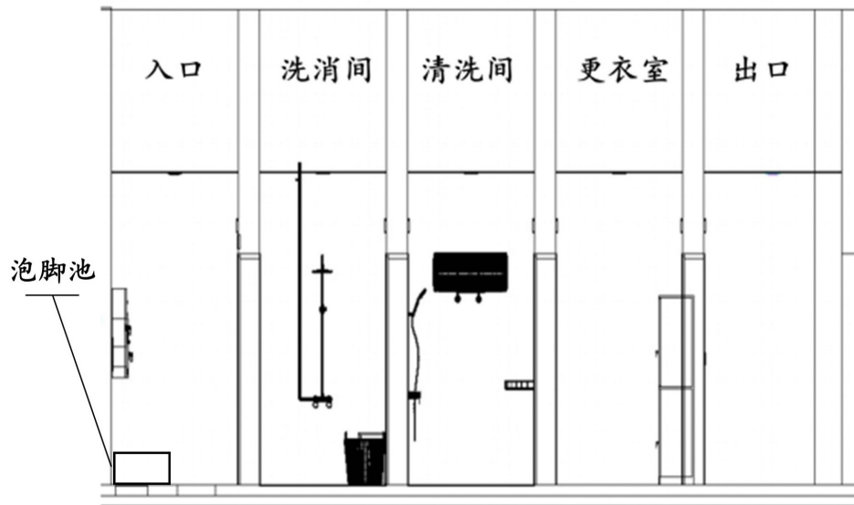
图 A. 2 救援人员洗消单元模式图
