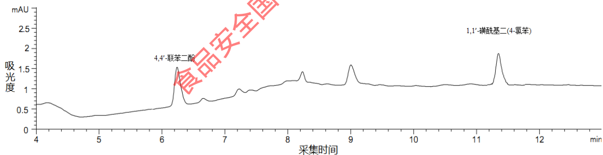
图 A.3 异辛烷中 4,4'-联苯二酚和 1,1'-磺酰基二(4-氯苯)标准溶液 (0.050 mg/L) 液相色谱图
