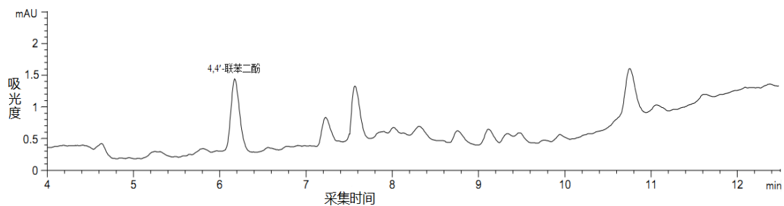
图 A.4 玉米油食品模拟物中 4,4'-联苯二酚标准溶液 (0.050 mg/kg) 液相色谱图
