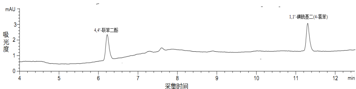
图 A.1 乙腈-水溶液 (1+1) 中 4,4'-联苯二酚和 1,1'-磺酰基二(4-氯苯)标准溶液 (0.050 mg/L) 液相色谱图
