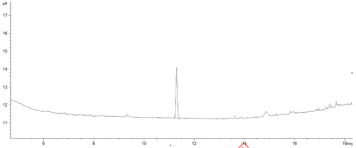
图 B 二苯醚标准溶液的气相色谱图（浓度为 0.05 \mu\text{g}/\text{mL} ）
