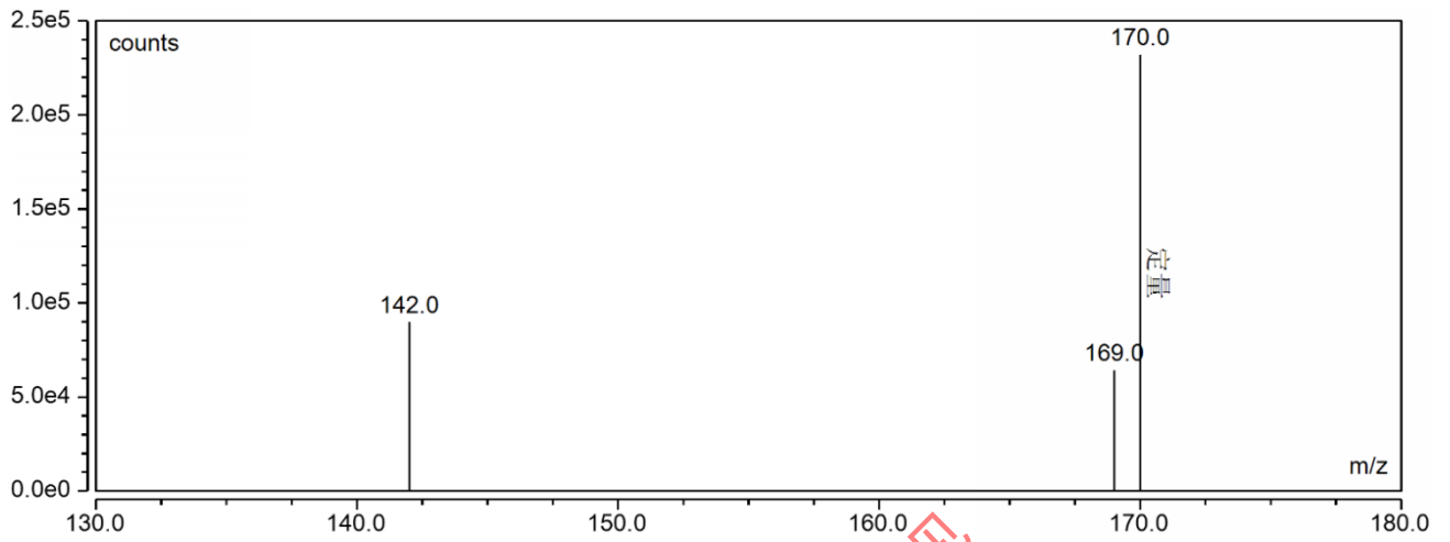
图 A.1 二苯醚标准溶液的质谱图
