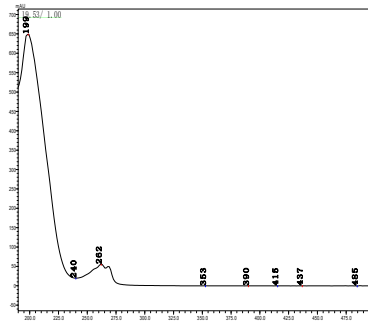
粉唑醇
