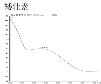
甲基咪草烟
