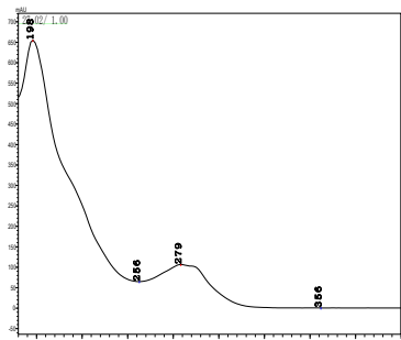
氟虫腈
