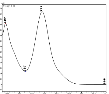
嘧霉胺
