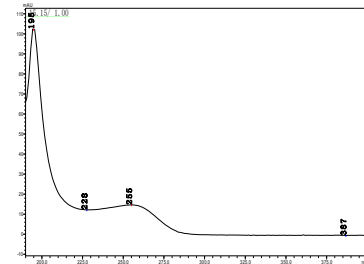
苯磺隆
