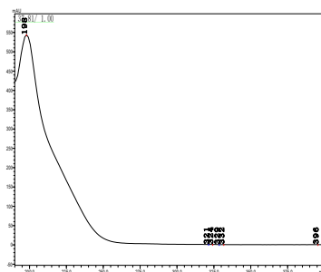
氯烯炔菊酯
