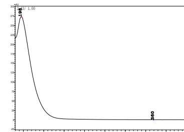
双丙胺磷钠
