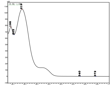
莠去津
