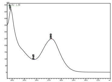
氰霜唑
