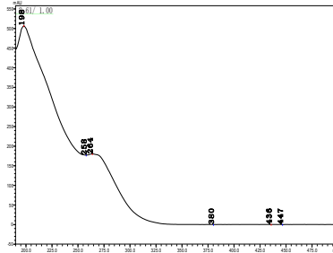
咪唑烟酸
