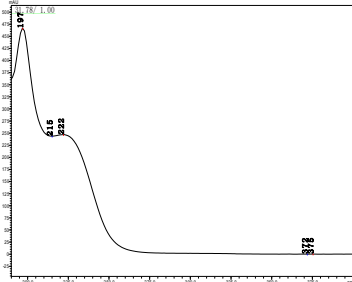
炔丙菊酯
