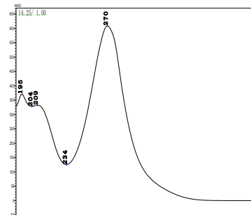
吡虫啉
