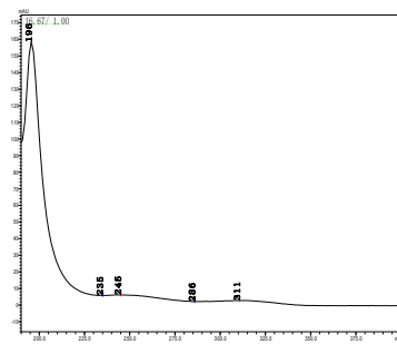
溴敌隆
