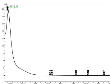
印楝素 II
