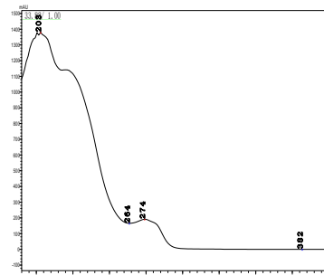
氰戊菊酯
