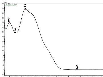
啉啉磺隆
