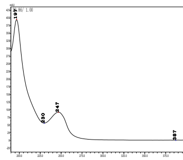
二嗪农
