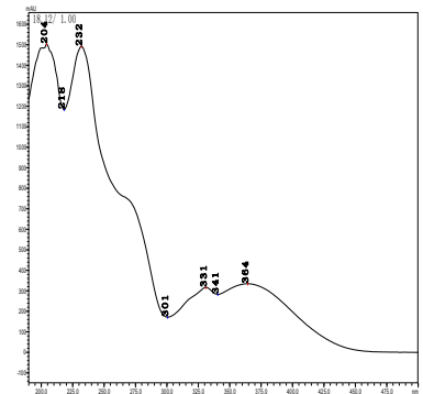
三氯苯嘧啶
