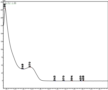
苯嘧磺草胺
