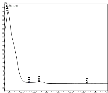
异丙威
