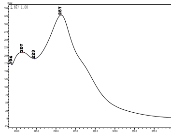
硝磺草酮
