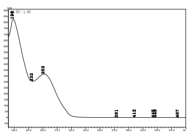
氟酰胺
