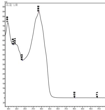
烯炔菌酯
