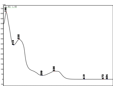
喹禾糖酯
