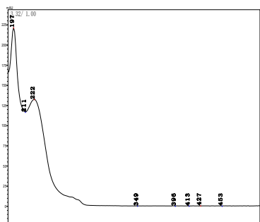
苯甲酸
