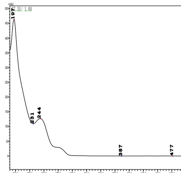
唑草酮
