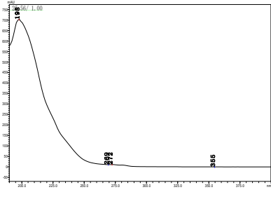
腐霉利
