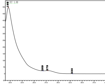
甲氧虫酰肼
