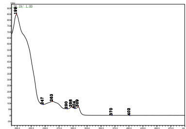
啶螨醚
