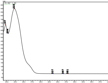
特丁净
