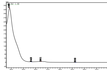
仲丁威
