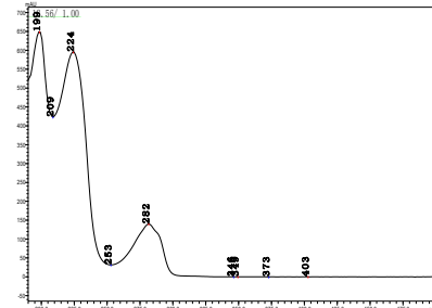
对氯苯酚
