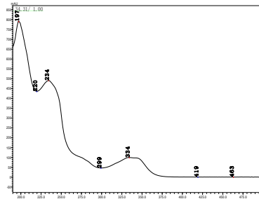
噁草酸
