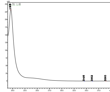
单甲脒
