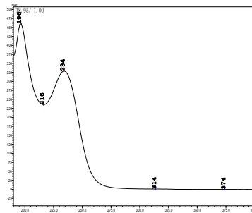
拉维因
