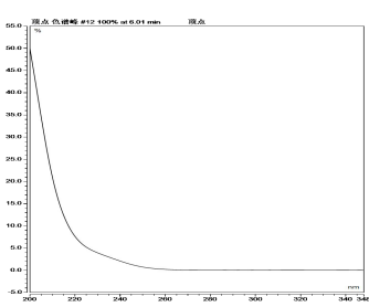
异乐果
