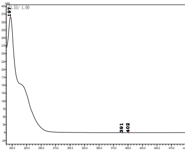
硫丹醚
