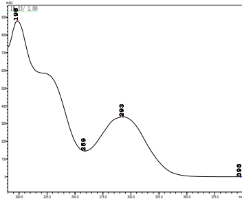
啉草酮
