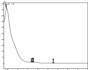
甲草胺
