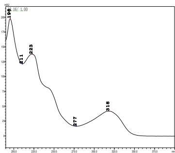
噻霉酮
