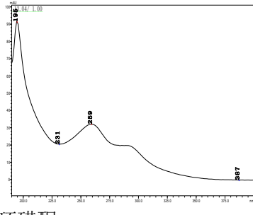
环磺酮
