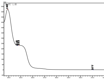
三氯杀螨醇
