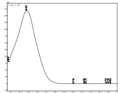
(+)-脱落酸
