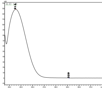
久效磷
