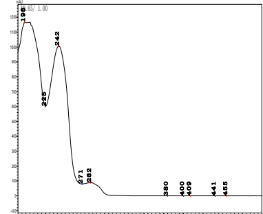
绿麦隆
