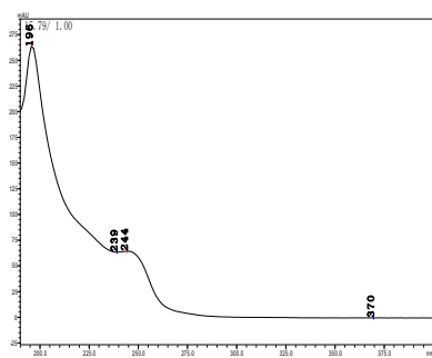
双草醚
