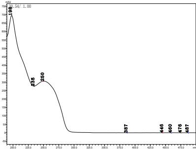
噻螨酯
