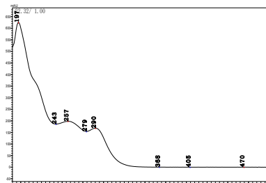
解草酮
