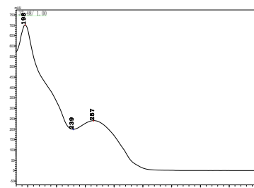
氟啉脲
