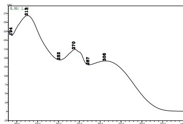
烯啶虫胺
