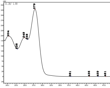
棉隆
