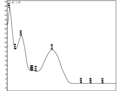
双丙环虫酯
