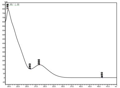
苯菌酮
