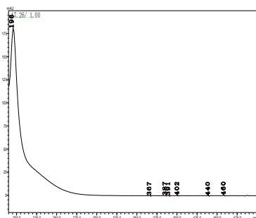
溴菌腈
