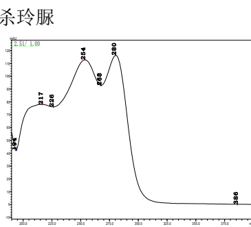
福美肿 I
