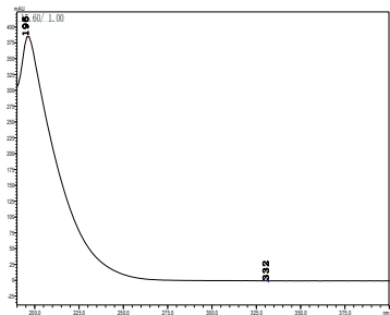
乐果
