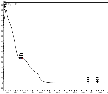
氟酰胺
