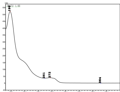
乙啉啉
