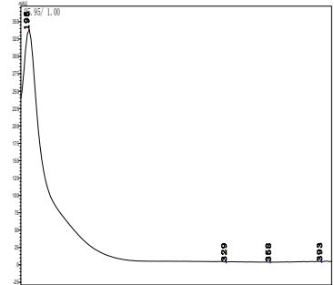
马拉硫磷
