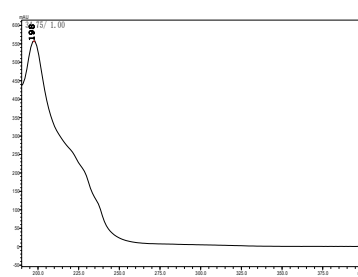
胺菊酯
