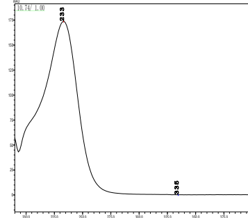
灭多威
