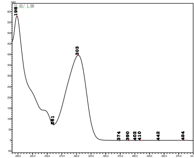
丙酯草醚
