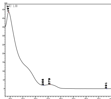
异丙胺
