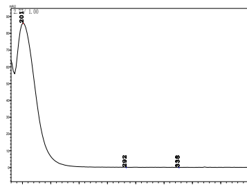
赤霉素(酸)
