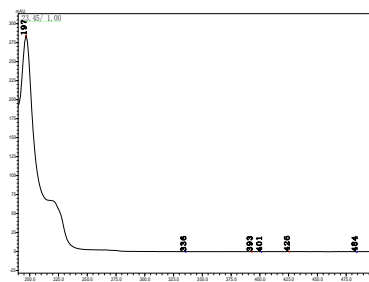
环唑醇
