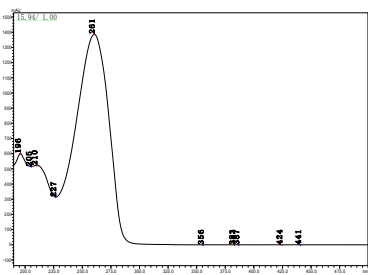
氟吡呋喃酮
