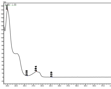
2.4 滴二甲铵盐
