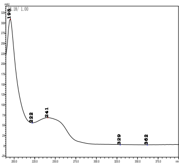
甲基二磺隆
