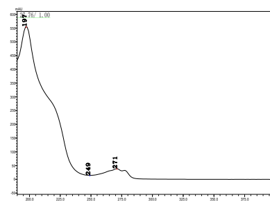
苯硫威
