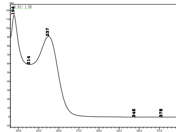
盐酸吗啉胍
