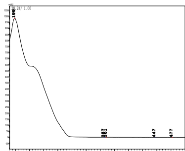
氟丙菊酯
