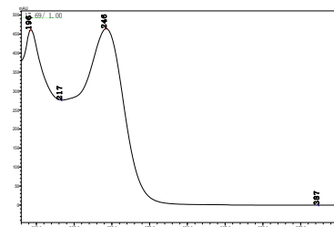
环啉酮
