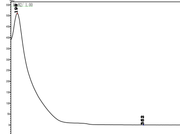
氯菊酯
