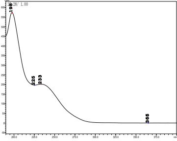
虫酰肼
