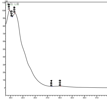
五氯硝基苯
