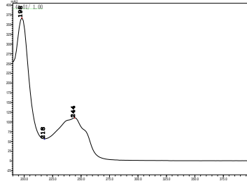
阿维菌素
