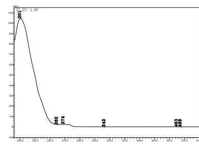
乙烯菌核利
