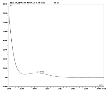
杀虫单
