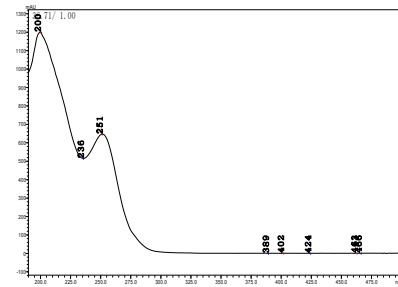
丁醚脲
