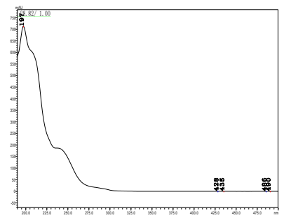
苯酰锰锌
