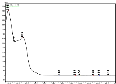
戊菌隆
