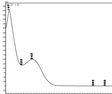
三唑磷
