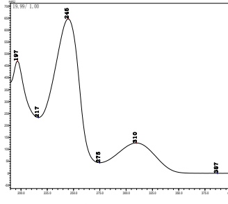
抗蚜威
