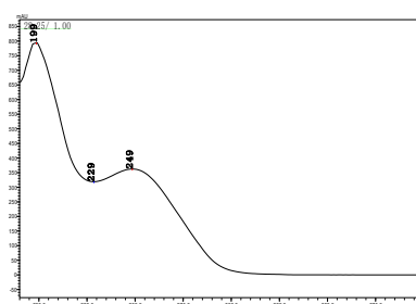
杀铃脲
