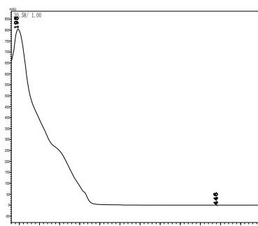
苯醚菊酯
