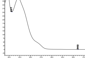
莠灭净
