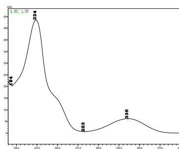
灭草松
