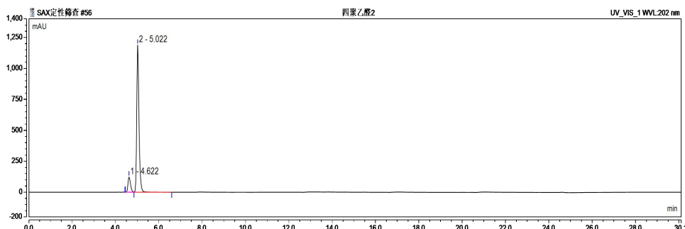
图1 四聚乙醛和内标物的典型高效液相色谱图
