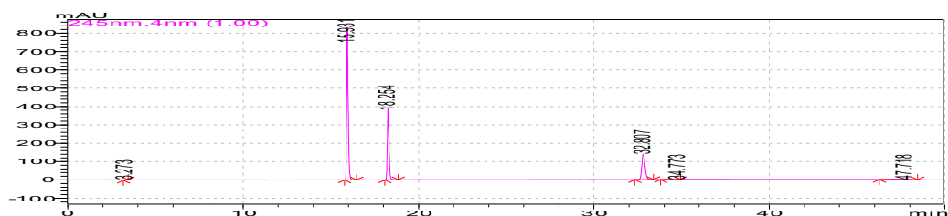
图1 氟吡呋喃酮-内标物的典型高效液相图
