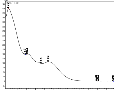
苯唑草酮
