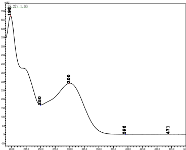
乙唑螨腈
