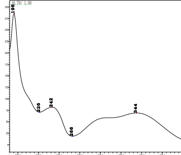
复硝酚钠
