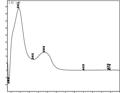
啶磺草胺
