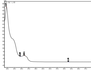
啶菌噁唑
