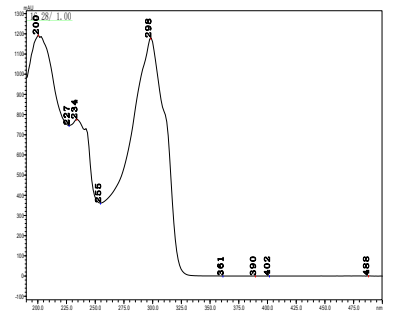
噻菌灵
