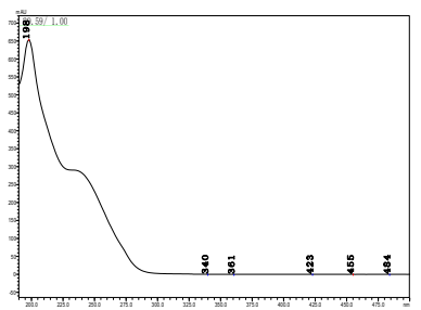
环氟菌胺
