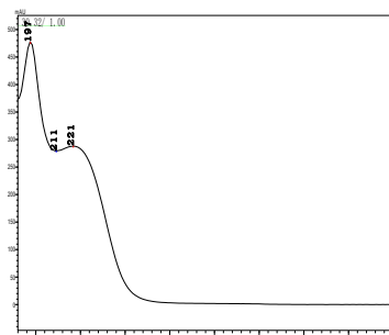
氯丙炔菊酯
