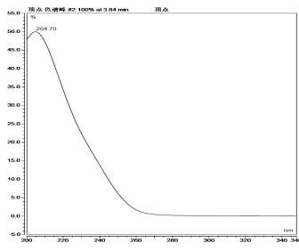
春雷霉素
