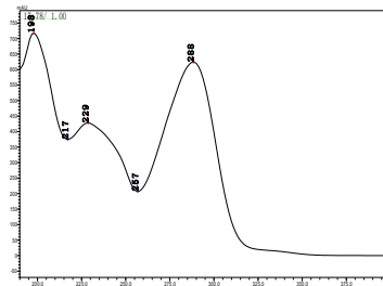
噻苯隆
