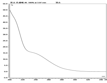
单甲脒 II
