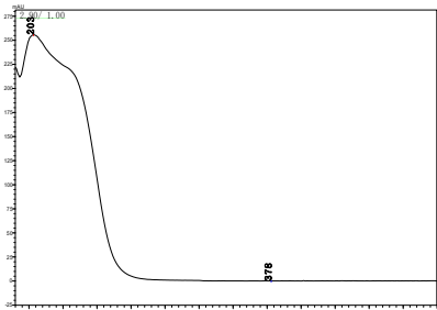
噻酮磺隆
