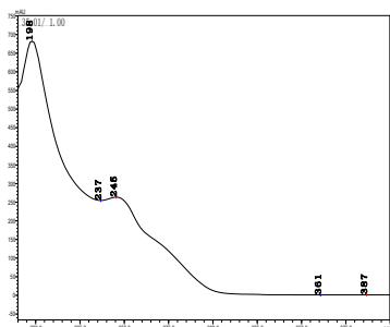
啉啉草醚
