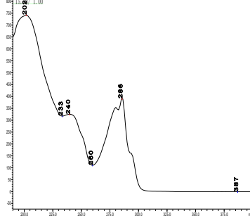
多菌灵
