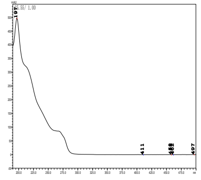
氟醚菌酰胺
