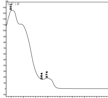
溴氰菊酯
