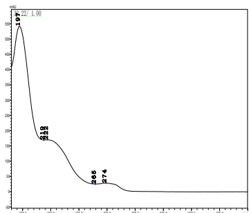
鱼藤酮
