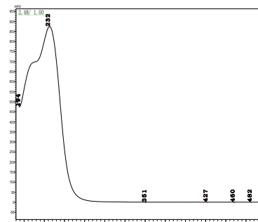
乙撑硫脲
