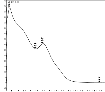
甲基硫菌灵
