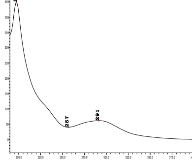
乙羧氟草醚
