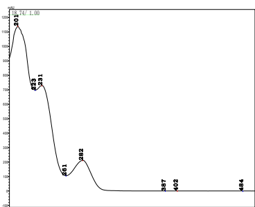
2,6-二甲基苯胺
