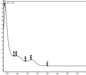
甲基二磺隆
