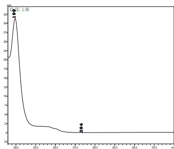
松脂酸铜
