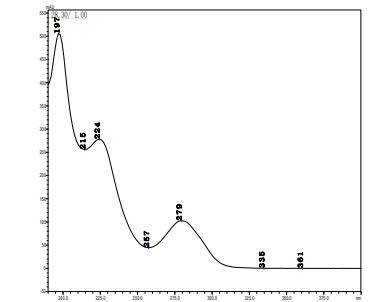
炔草酯
