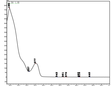
噁虫酮
