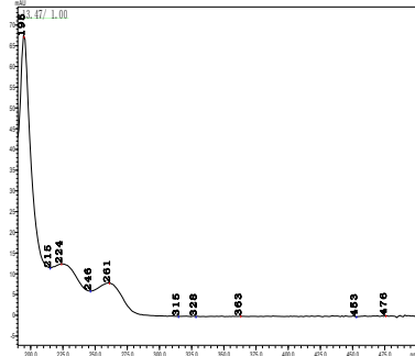
二氟苄腈
