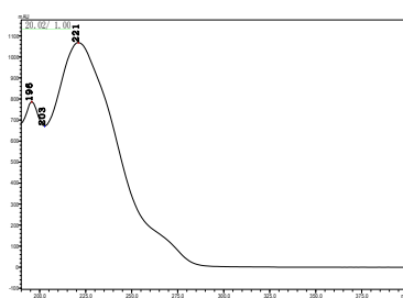
西草净
