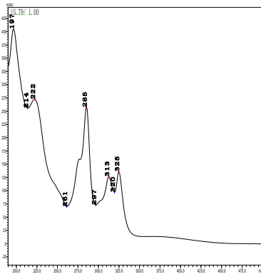
氯鼠酮
