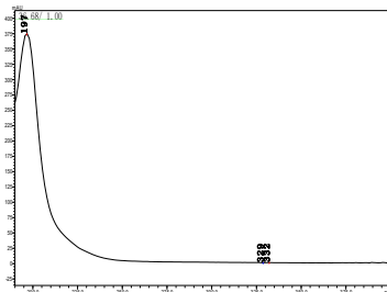
硫丹
