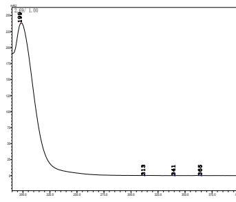
丙烯酸
