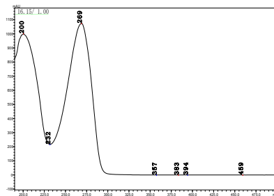
卞氨基唑啉
