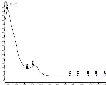
乙虫腈
