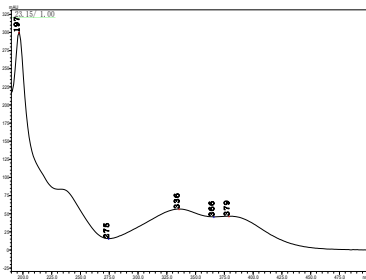
杀螺胺
