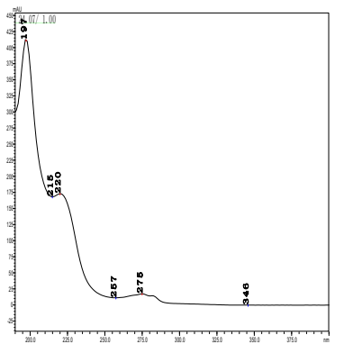
三啉酮
