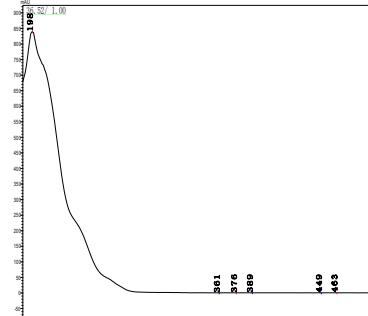
氟草烟酯
