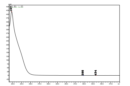
禾草敌
