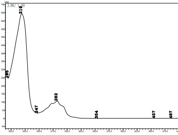
萘乙酸钠
