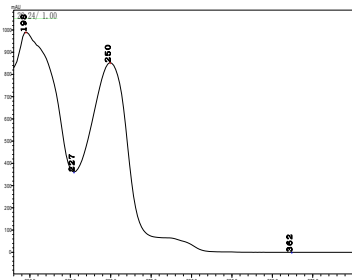
敌草隆
