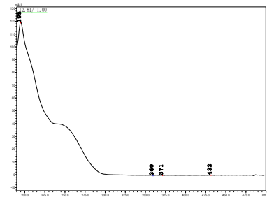
双氯磺草胺
