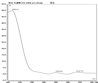
胺鲜酯
