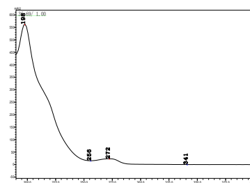
氯氟醚菊酯
