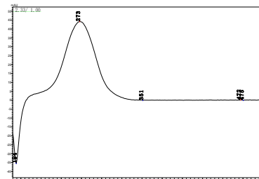
调环酸钙盐
