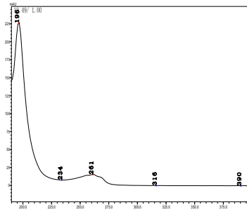
烟碱
