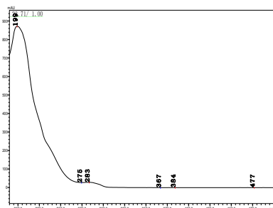
炔苯酰草胺
