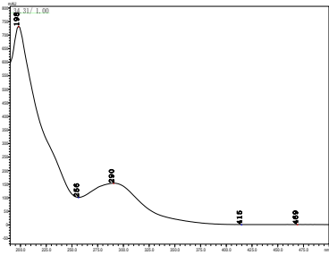
乳氟禾草灵
