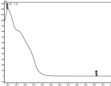
烟酰胺
