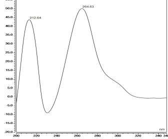
灭蚁灵
