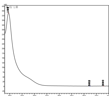
特丁硫磷
