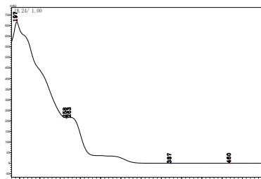
甲磺草胺
