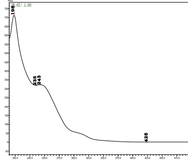
硝苯菌酯
