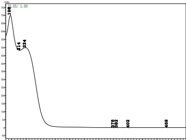
烯丙菊酯
