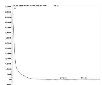
矮壮素
