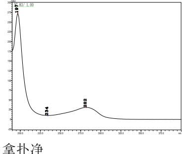
拿扑净
