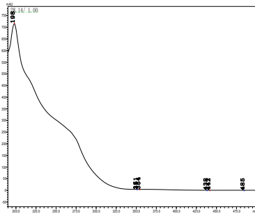
SP-1
