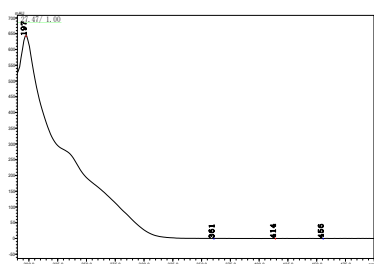
氟苯虫酰胺
