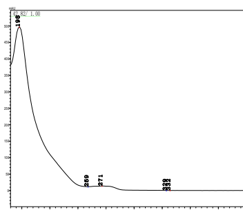
苯醚菊酯
