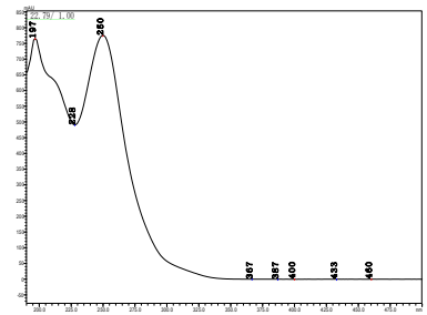
氟氯吡啶酯
