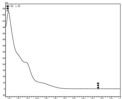
酰胺唑
