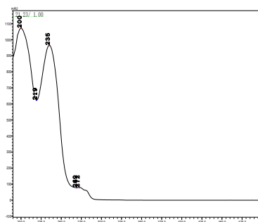
甜菜宁
