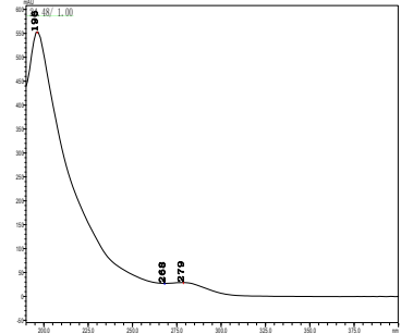
甲氧虫酰肼
