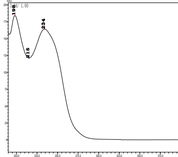
甲磺隆
