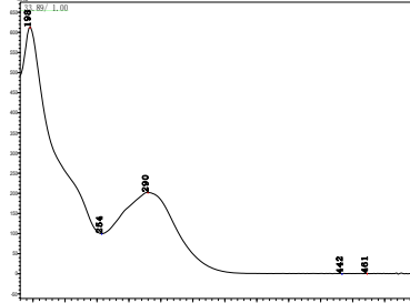
氟吡草胺
