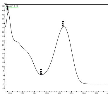
噻唑菌胺
