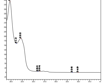
对-二氯苯
