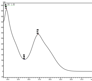
哒优麦
