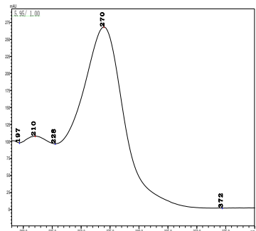
呋虫胺
