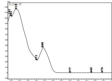
丙硫多菌灵
