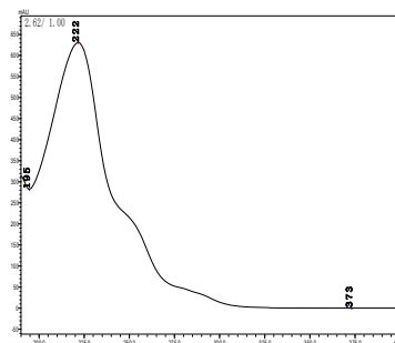
氨基吡啶酸
