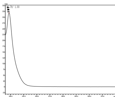
氯吡磷
