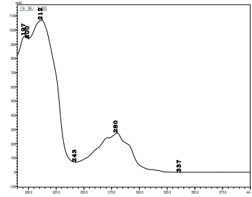
甲萘威
