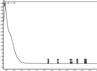
硫丹醇
