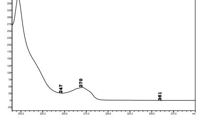
氟吡菌酰胺
