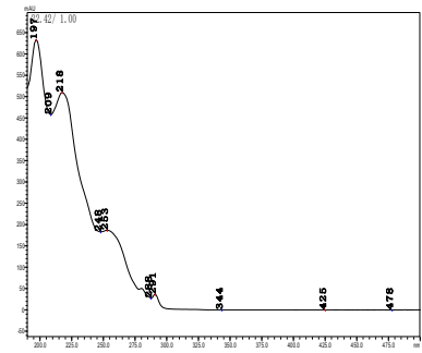
氟菌唑
