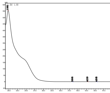
氟硫草定
