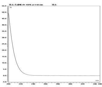
敌百虫
