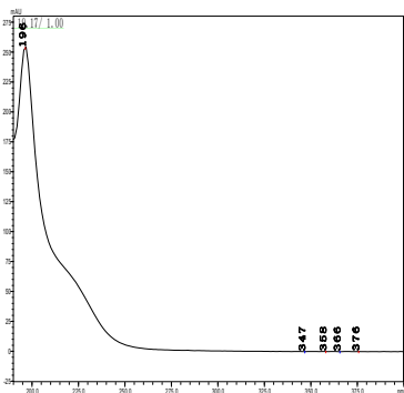
印楝素 I
