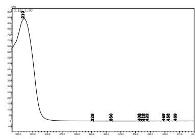
单氰胺
