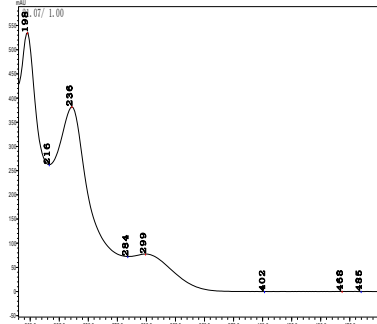
环酰菌胺
