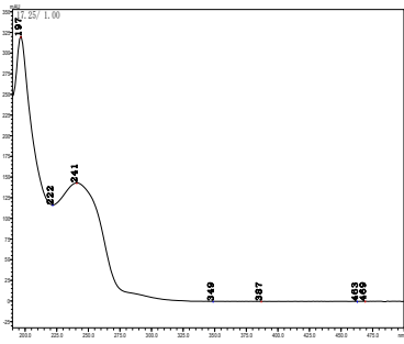
啉苯胺磺隆 2
