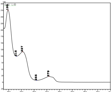
二甲四氯
