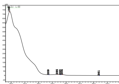
辛酰溴苯腈
