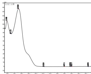
单嘧磺酯
