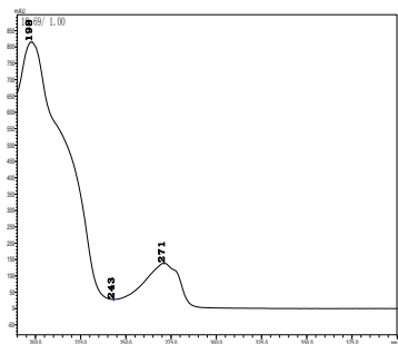
残杀威
