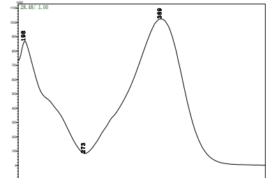
补骨脂乙素
