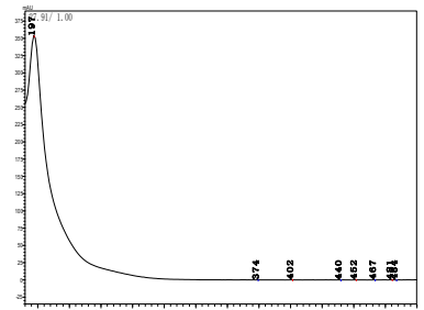
大蒜素
