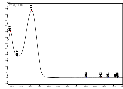
丁噻隆
