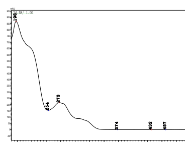
氟啶唑
