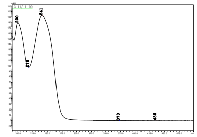
酰嘧磺隆
