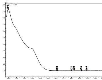
普施特
