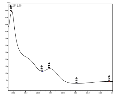
氟乐灵
