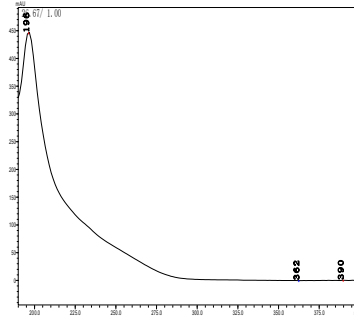
噻呋酰胺
