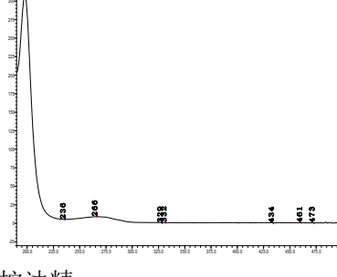
桉油精
