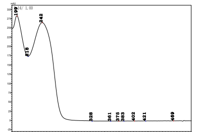
四啞啞磺隆
