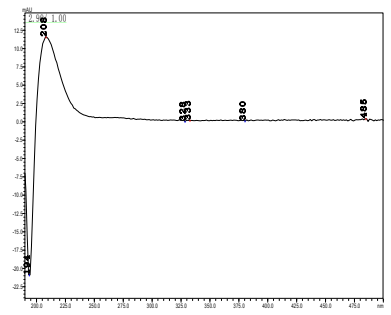
氯化钠
