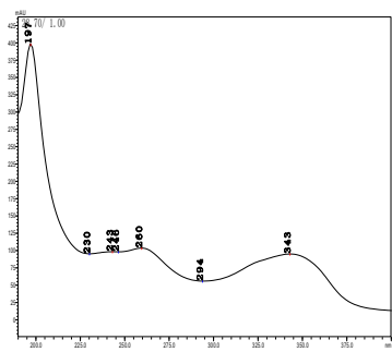
氟啶胺
