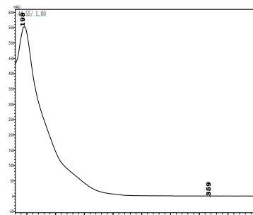
联苯菊酯
