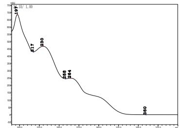
联苯肼酯
