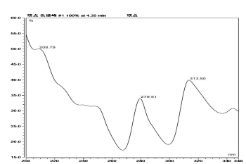
三乙膦酸铝
