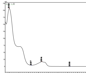
2,4-D 二甲胺
