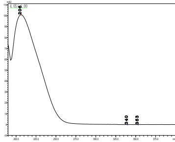
噁霉灵
