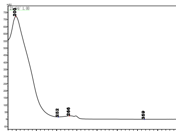
精甲霜灵
