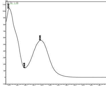
除草醚
