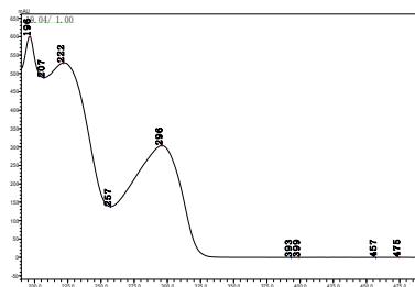
乙嘧酯
