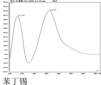
苯丁锡
