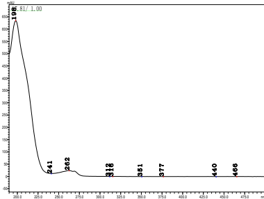
速灭威
