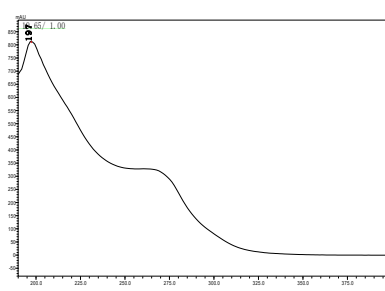
溴氰虫酰胺
