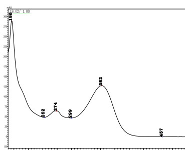
哌虫啉 2
