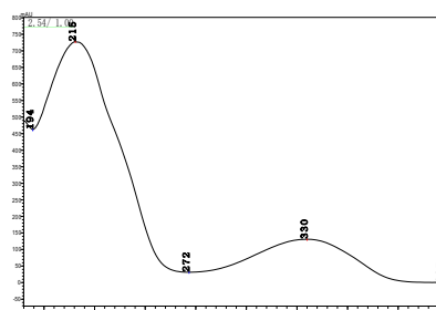
抑芽丹
