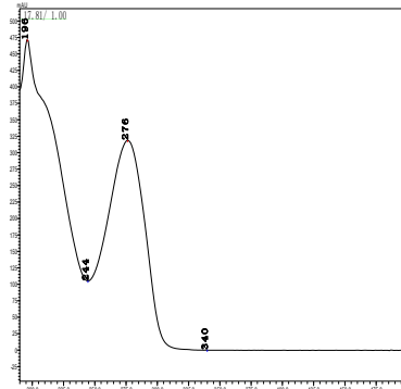
除草定
