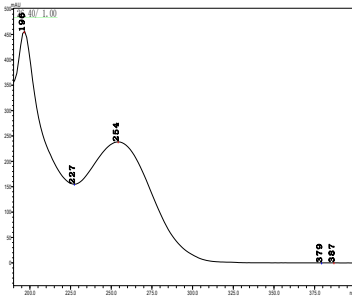
烯效唑
