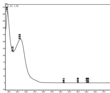
氟胺磺隆
