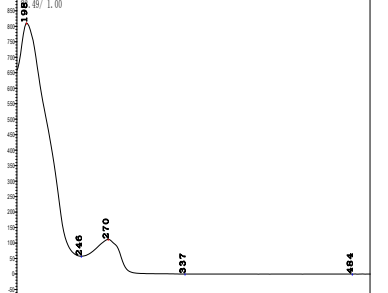
氟吡菌胺
