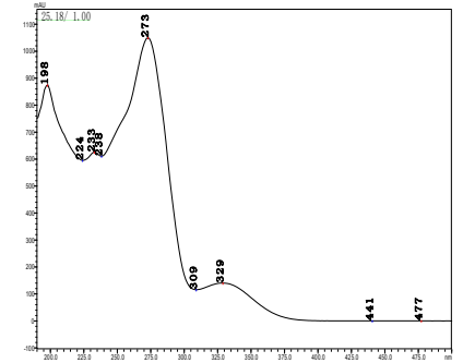
啉菌胺
