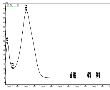
硫环磷
