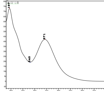
四螨嗪
