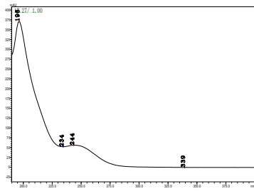
涕灭威
