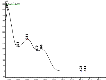
萎锈灵
