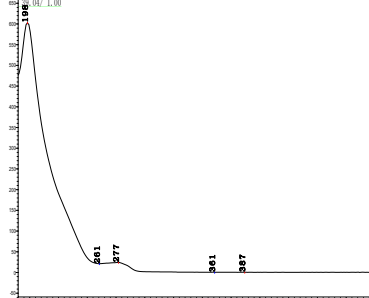
苯氟菊酯
