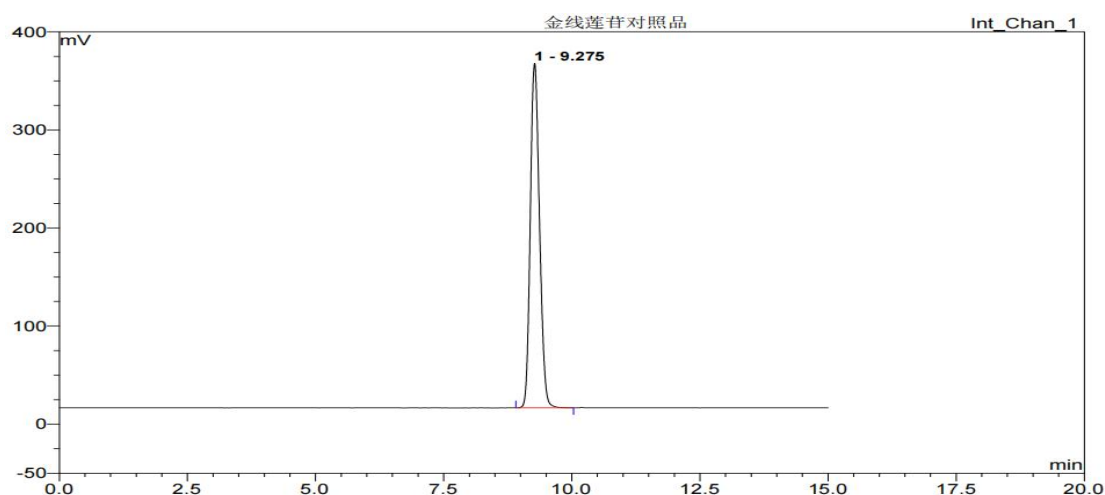
图 A. 1 金线莲苷对照品液相色谱图
