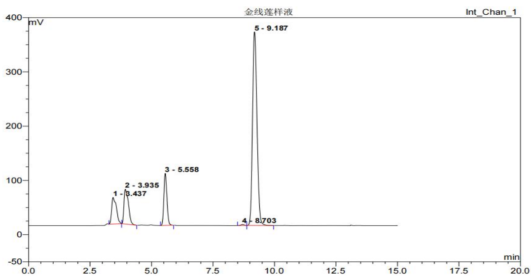
图 A. 2 金线莲样液液相色谱图
