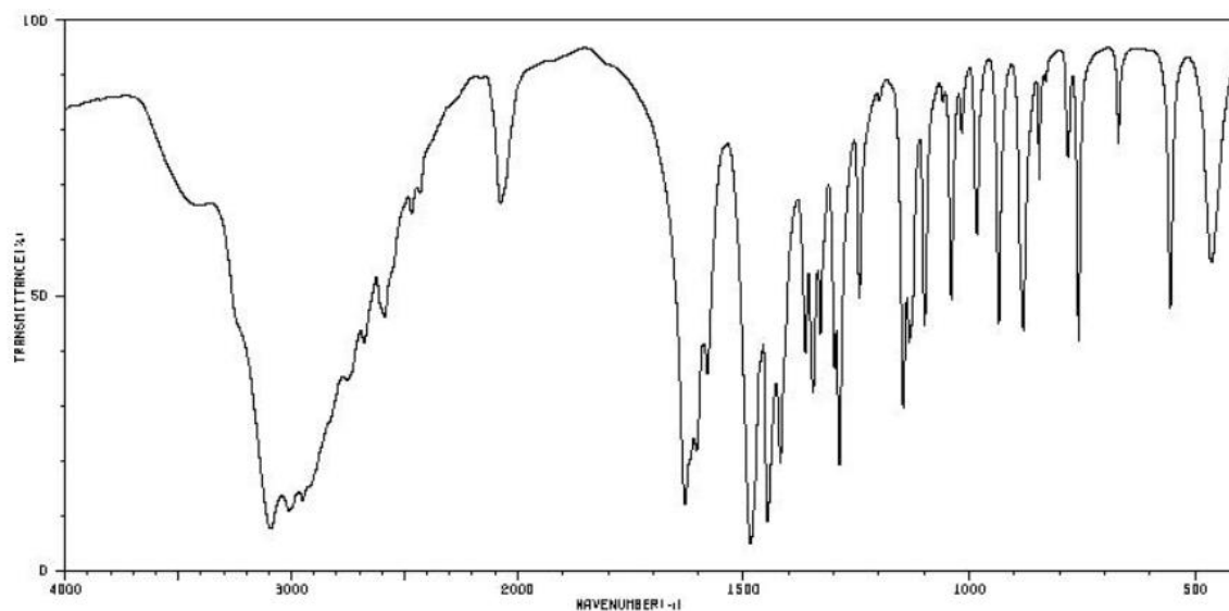
图 B.1 L-盐酸鸟氨酸标准品红外吸收光谱图
