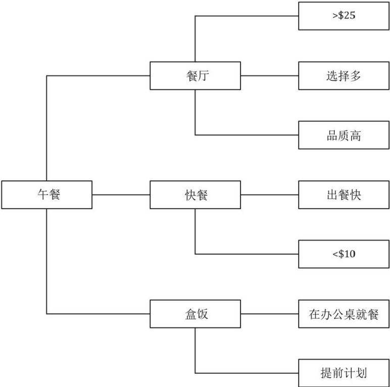
图 14 决策树
