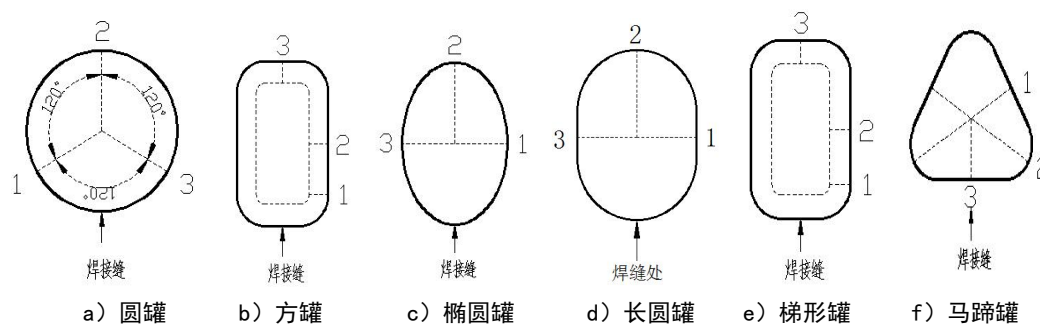
图 10 检测部位
