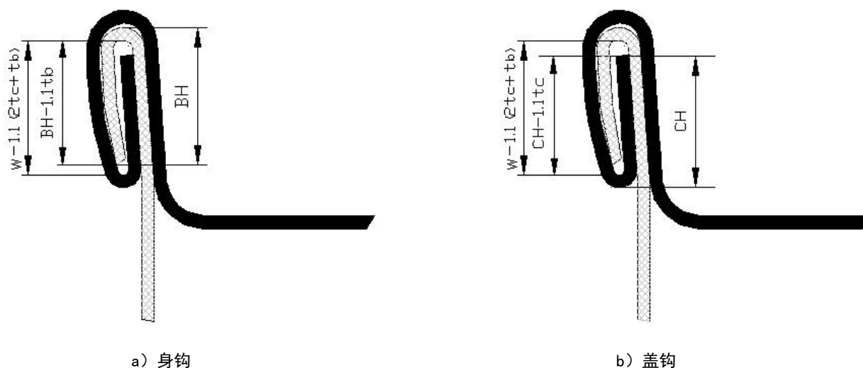
图 12 身钩和盖钩测量示意图
