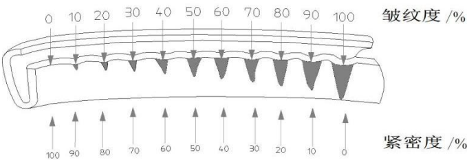
图 2 皱纹度和紧密度
