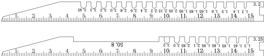
图 8 罐头工业专用卡尺
