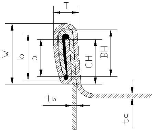
图 D.1 二重卷封测量示意图
