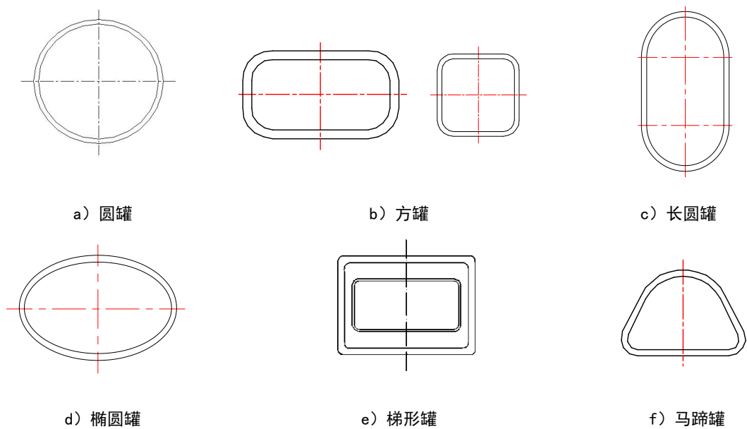
图5 圆罐和异形罐横截面示意图
