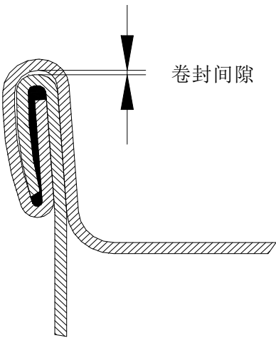
图 3 卷封间隙
