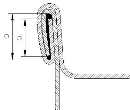
图 11 叠接长度和叠接率测量示意图
