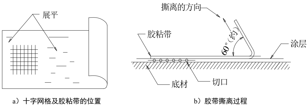
图 14 液体补涂附着力试验示意图
