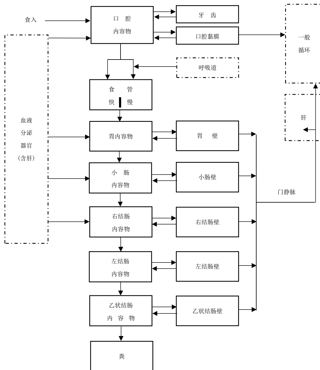
图 A.3 人消化道模型（HATM）的结构
